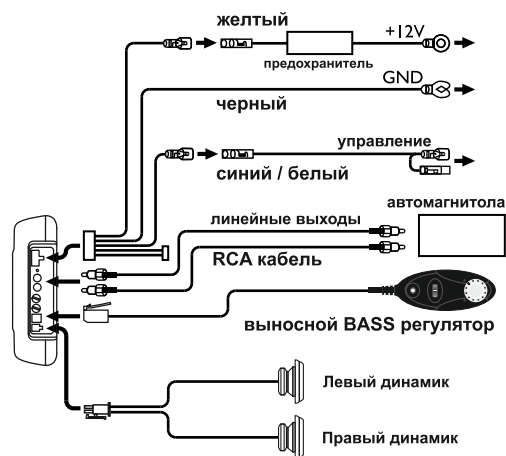
A. Схема подключения сабвуфера к головному устройству через НЧ линейные входы RCA
