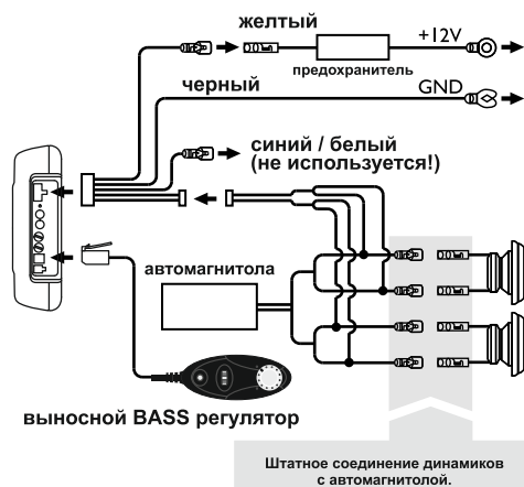
B. Схема подключения сабвуфера к головному устройству по высокоуровневым входам (к динамикам)
